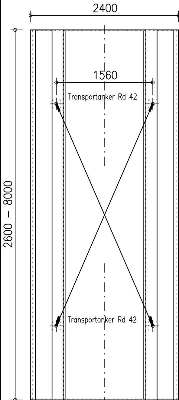
DRAUFSICHT
